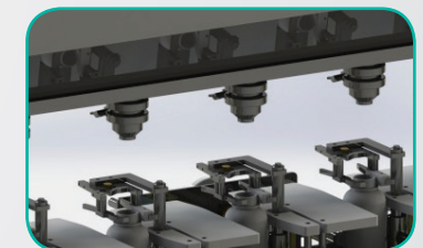
Bicos de envase com tecnologia anti pingos.
